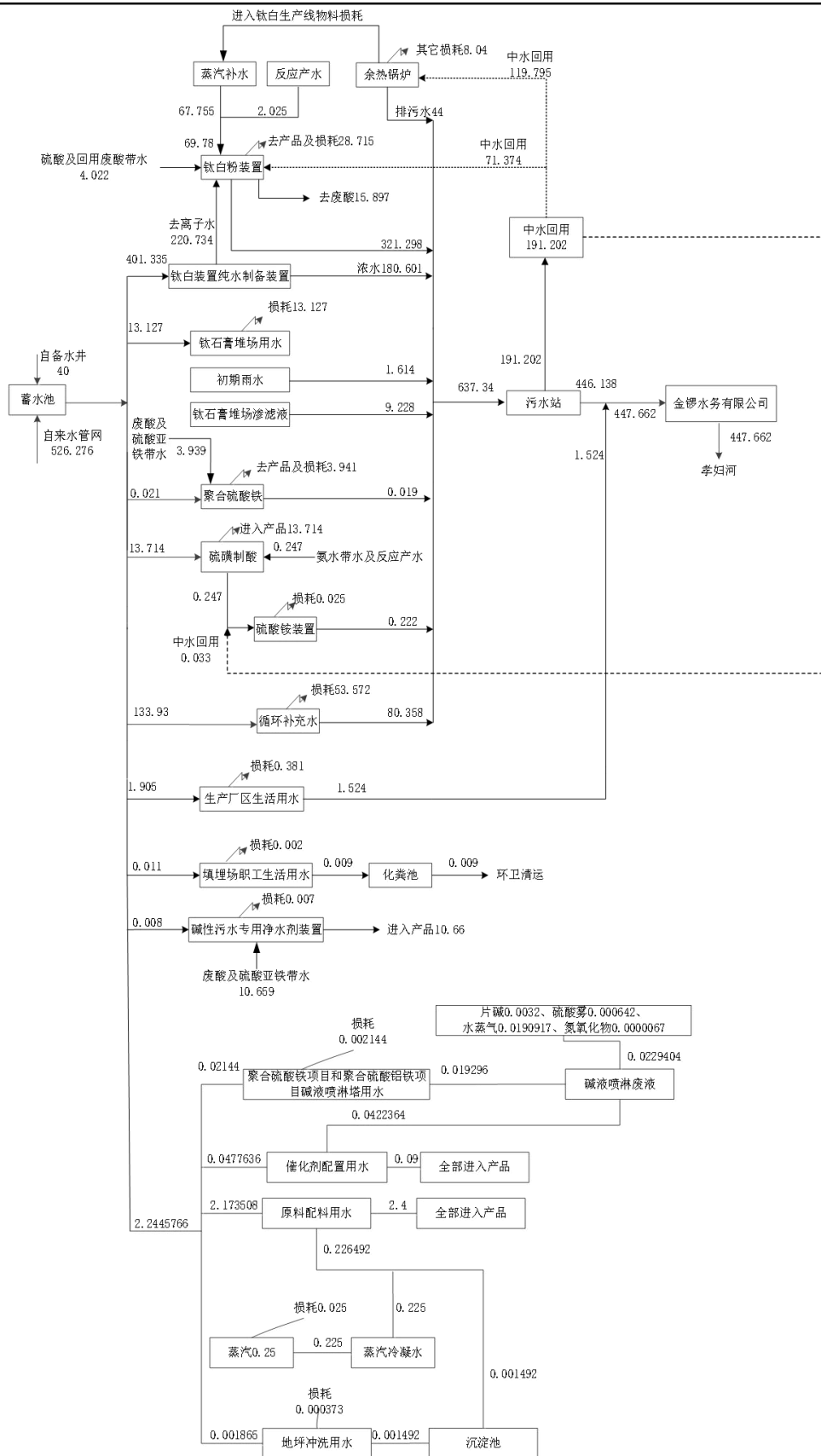
图 2-2 本项目建成后全厂水平衡图 (万 \text{m}^3/\text{a} )
