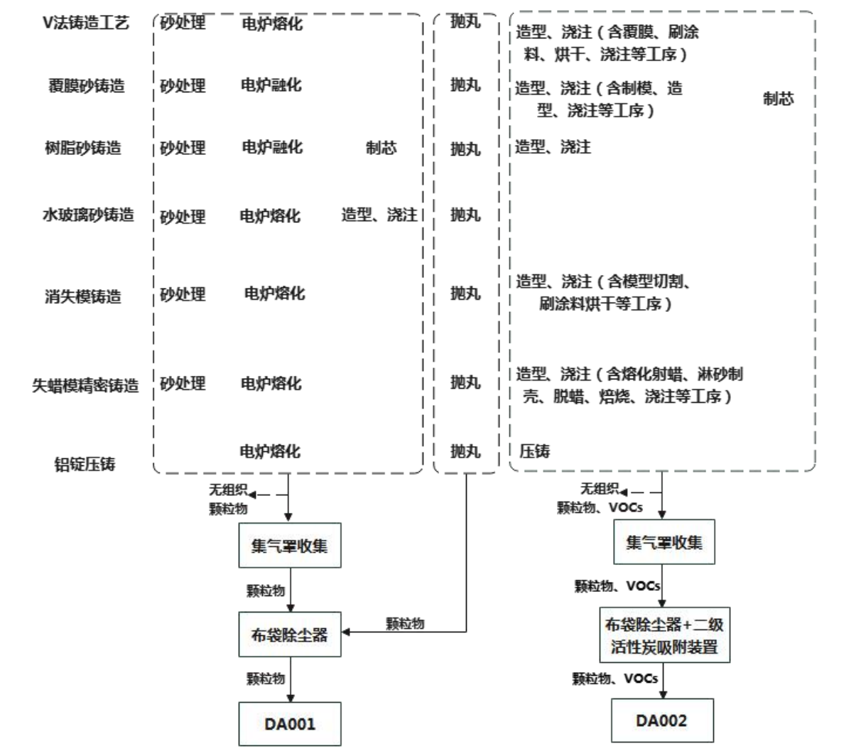
图 1-1 全厂废气走向图
