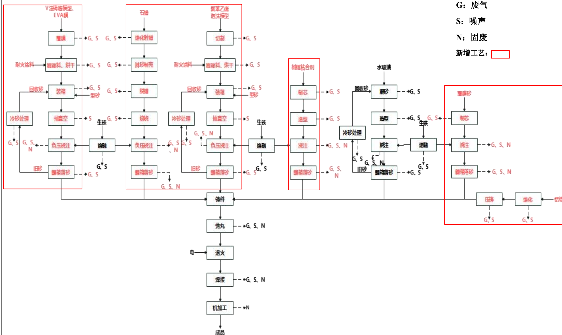
图 2-1 技改后项目水玻璃砂及新增 V 法铸造工艺、消失模精密铸造工艺、消失模铸造工艺、树脂砂铸造工艺、覆膜砂铸造工艺、铝合金压铸件工艺流程及产污节点图
