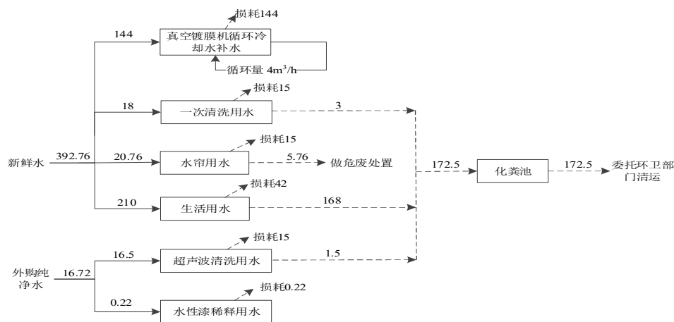
图 2 本项目水平衡图（单位 \text{m}^3/\text{a} ）
