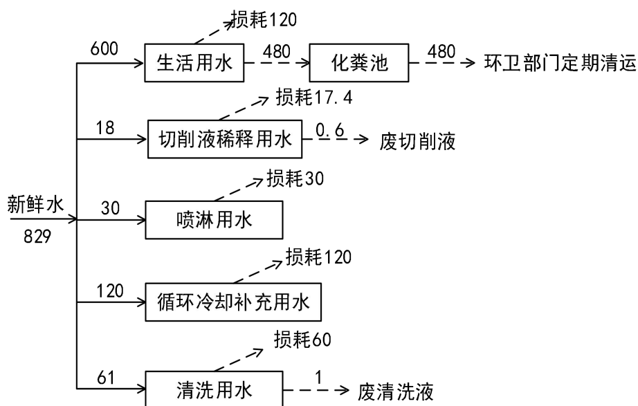
图 2-2 技改后全厂水平衡图（单位：m 3 /a）
