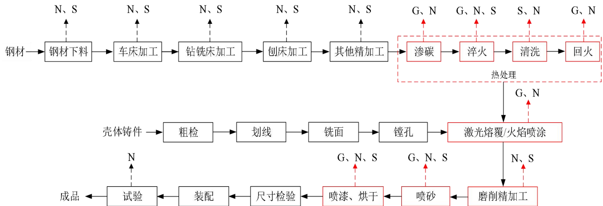
图 2-3 工艺流程及产污环节图
