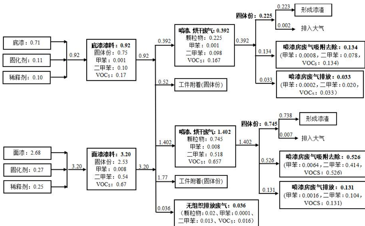
图 2-1 漆料平衡图 t/a
