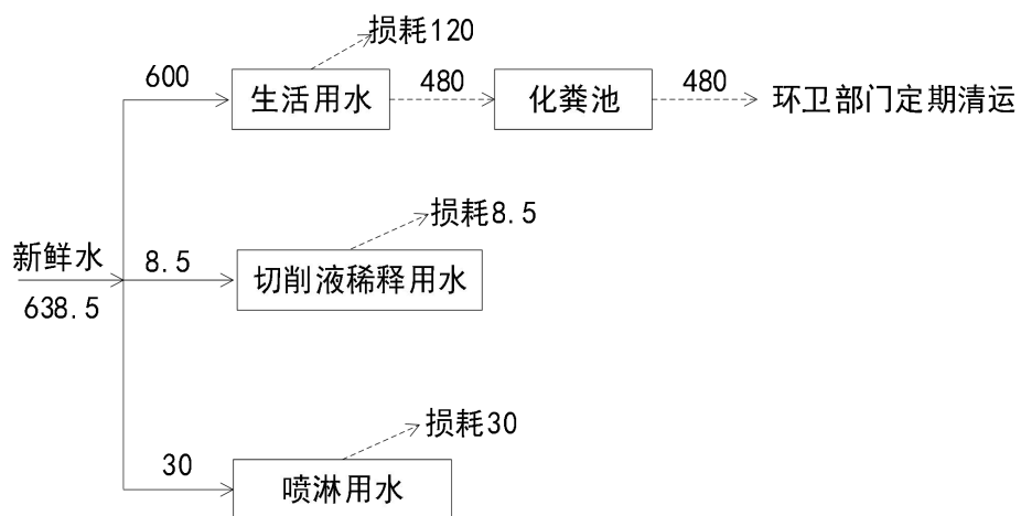
图 2-2 技改后全厂水平衡图（单位：m 3 /a）
