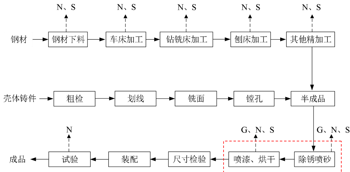
图 2-3 工艺流程及产污环节图
